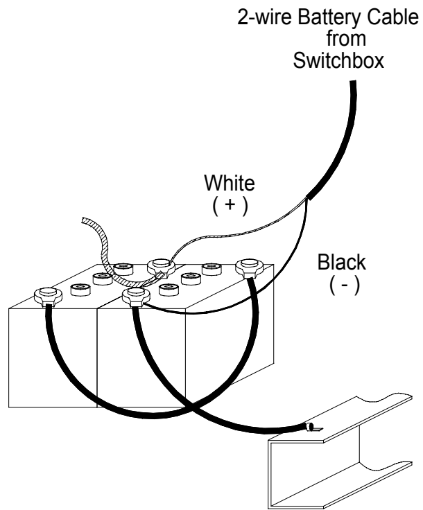
12 VOLT SYSTEM (Two 6 VOLT BATTERIES)
